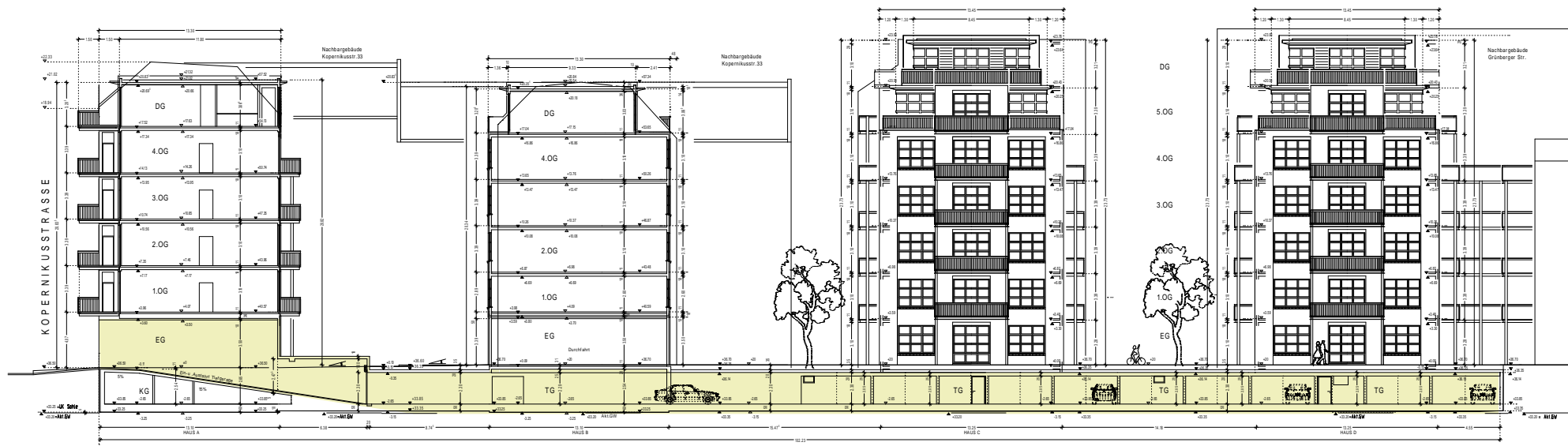
LOFTHOUSE A SCHNITT A-A
